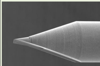
0.1φ 文字彫り用彫刻刃
