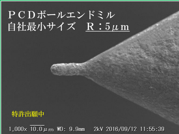
超微細PCD工具
