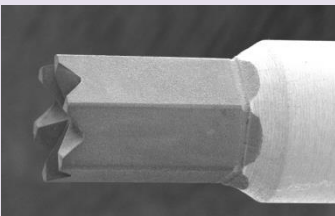
1.0φ PCDマイクロツール
